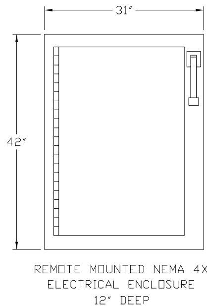
VIEW A-A
